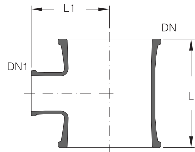
DN450 - DN1000
