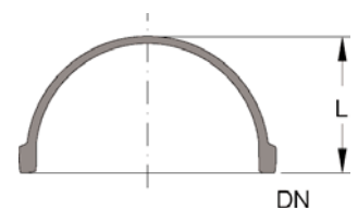
DN200 - DN300
