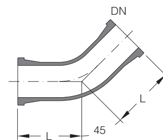
DN15 - DN100
